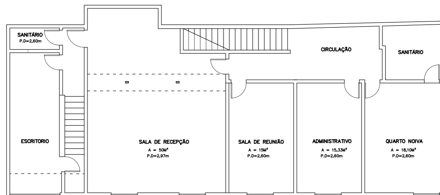
PLANTA – 1º PAVIMENTO SALÃO COMERCIAL ESCALA 1/100
