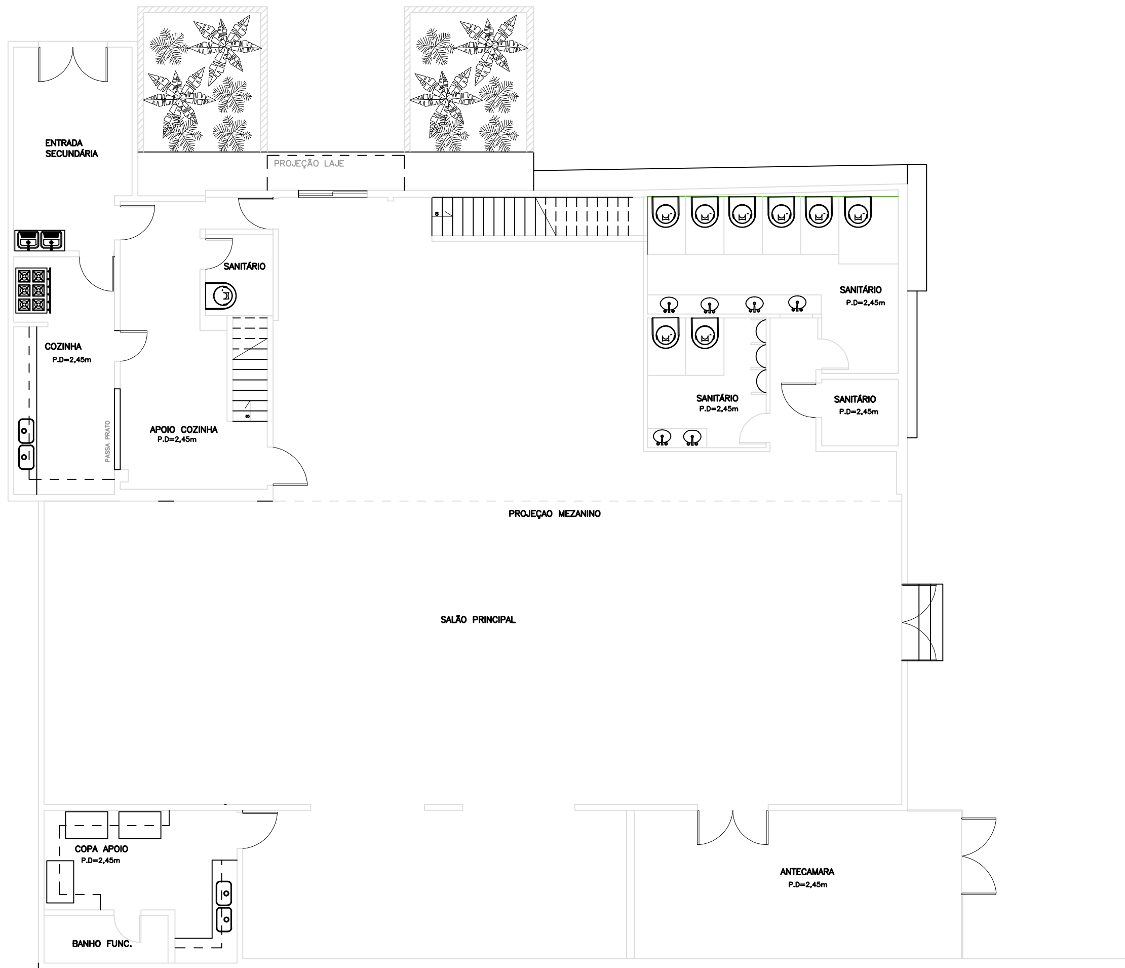
PLANTA LAYOUT TÉRREO SALÃO COMERCIAL ESCALA 1/100
